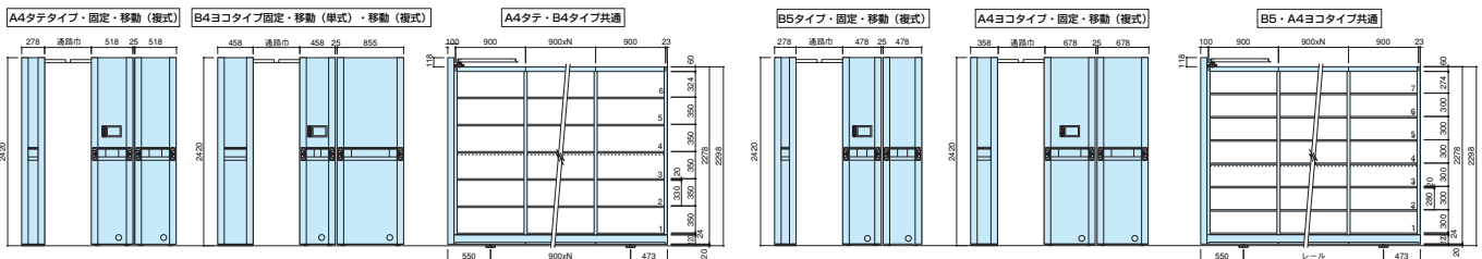
寸法図(mm)
