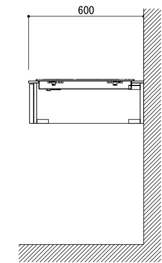
コンロ断面
