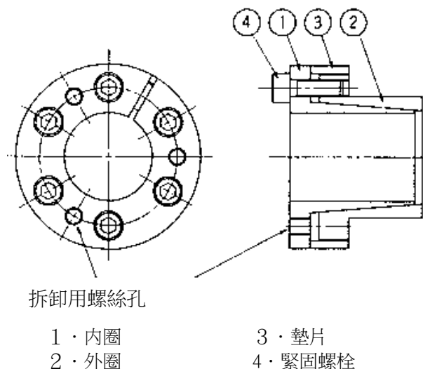
圖 1 零件名稱
