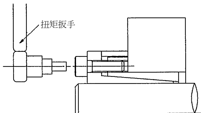
圖 2 安裝
