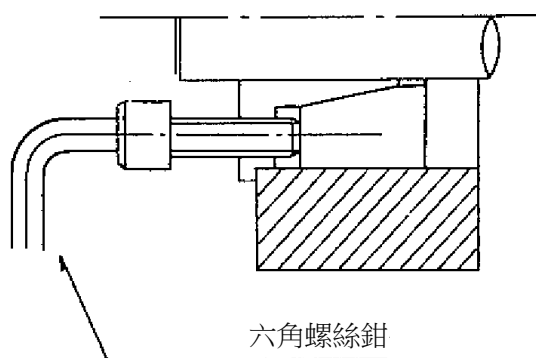
圖 4 拆卸
