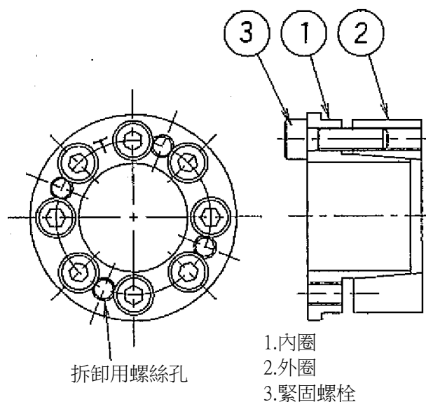
圖 1 零件名稱
