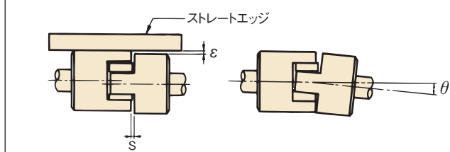
図3. 心出し図
