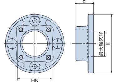
角ハブ
