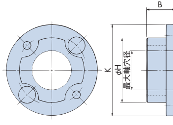
拡大ハブ
