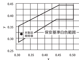
保安基準に規定されている色度範囲 '17年3月現在
