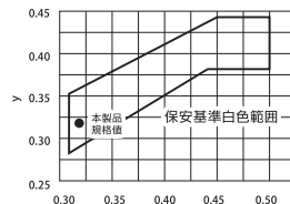
保安基準に規定されている色度範囲
