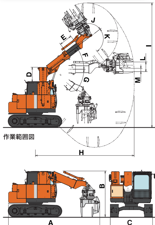
寸法図
