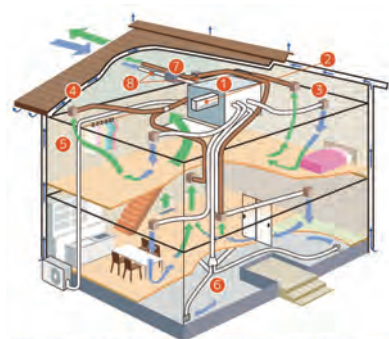
①空調室 (特許取得済) ②エアコン ③吹出グリル ④排気グリル ⑤コントローラー ⑥床下 ⑦熱交換気扇 ⑧フィルターボックス
