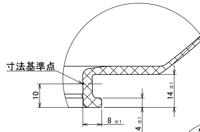
詳細図 A スケール 1 : 1
