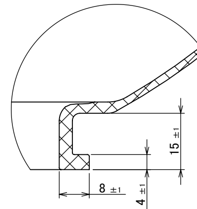
詳細図 A スケール 1:1
