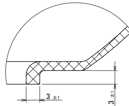
詳細図 A スケール 2 : 1
