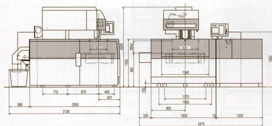
外形図
