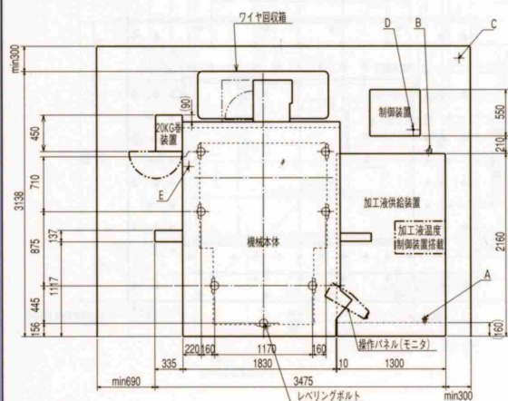
外形図
