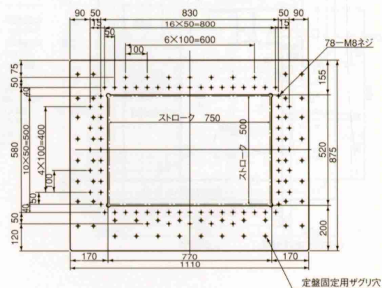
定盤図
