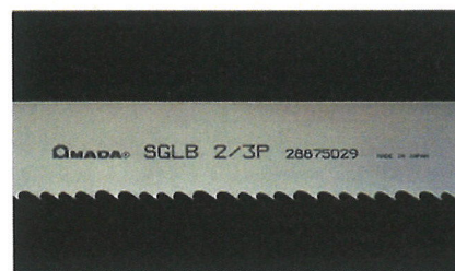
ブレード幅ワイド仕様
