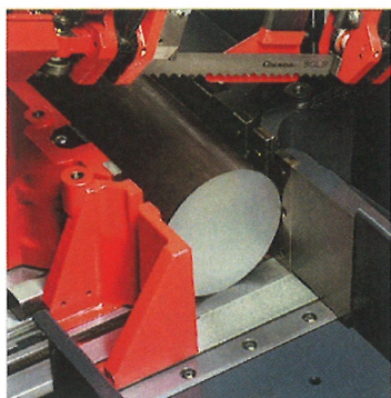
割りバイス構造 (HFA-250)
