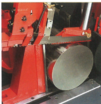
片側バイス構造 (HFA-400)
