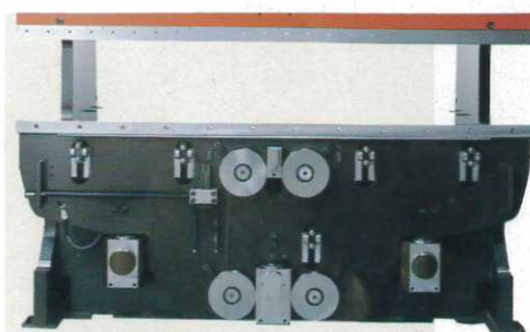
ローラーガイド (前後3~6カ所) ローラーガイド (左右)
