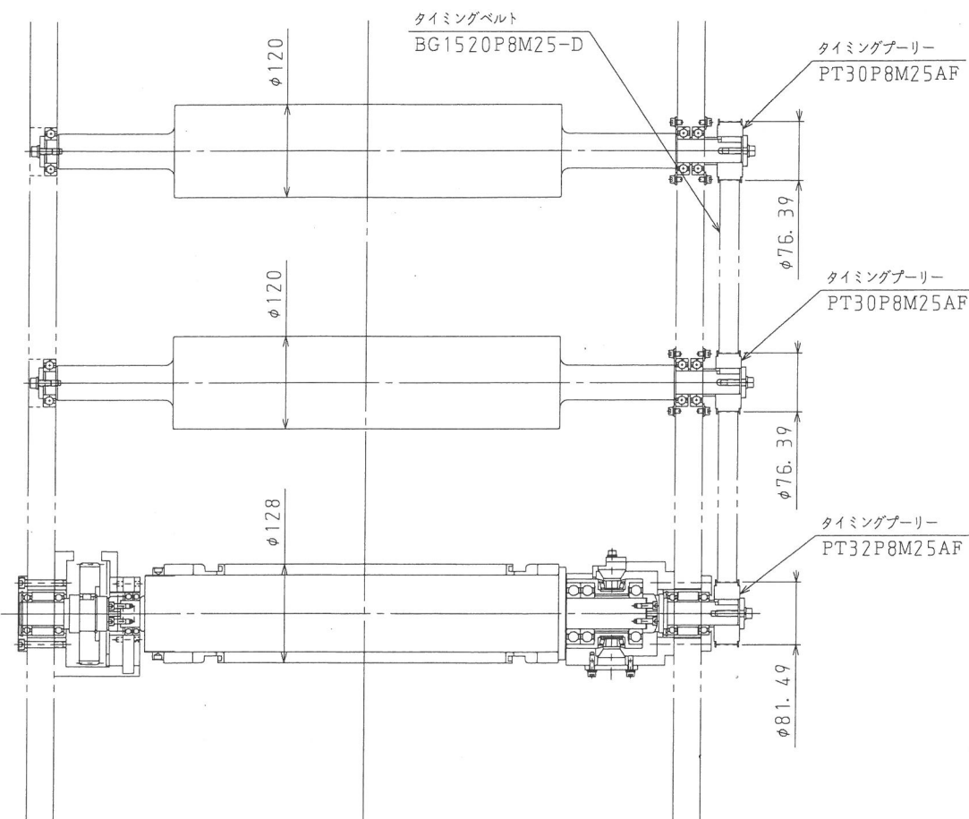
ライン駆動
