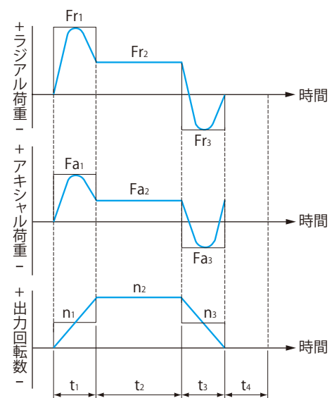
図 D6 変動荷重例
