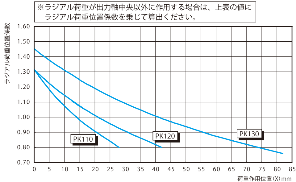
図 E2 ラジアル荷重位置係数
