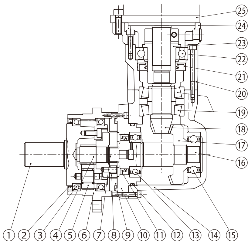
図E1 3段形 (例: ANFX-PK120N)
