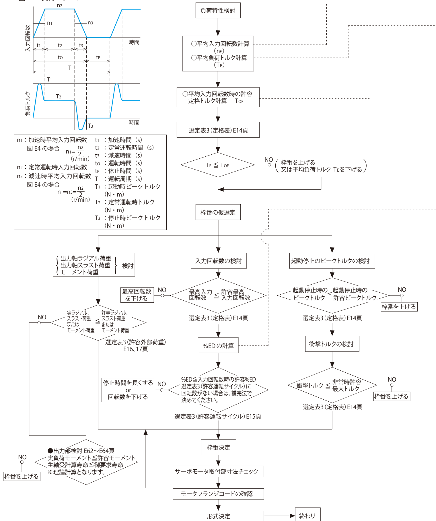
図 E4 負荷パターン
