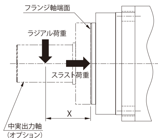
図D3 ラジアル荷重位置
