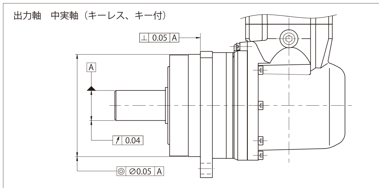
図 E7 中実軸機械的位置精度
