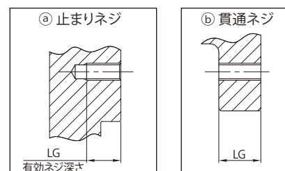
モーター取付ネジ形状詳細
