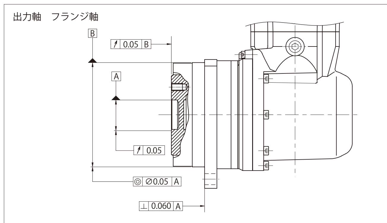
図 E8 フランジ軸機械的位置精度
