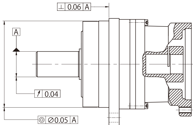
図 C7 中実軸機械的位置精度
