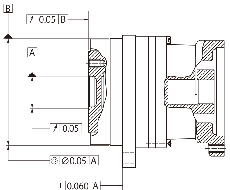
図 C8 フランジ軸機械的位置精度
