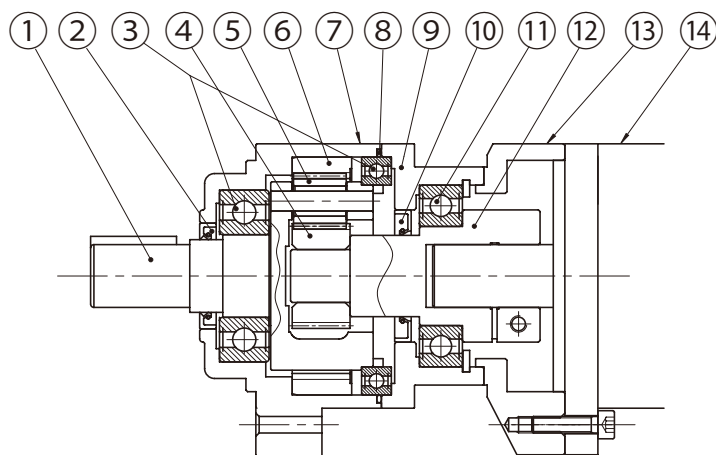
図B1 1段形 (例: ANFX-PE15W)
