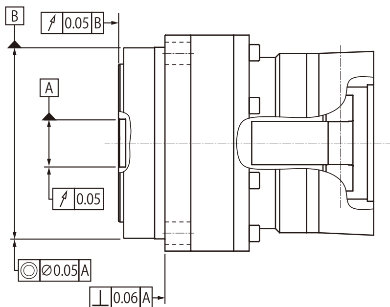
図 D8 フランジ軸機械的位置精度
