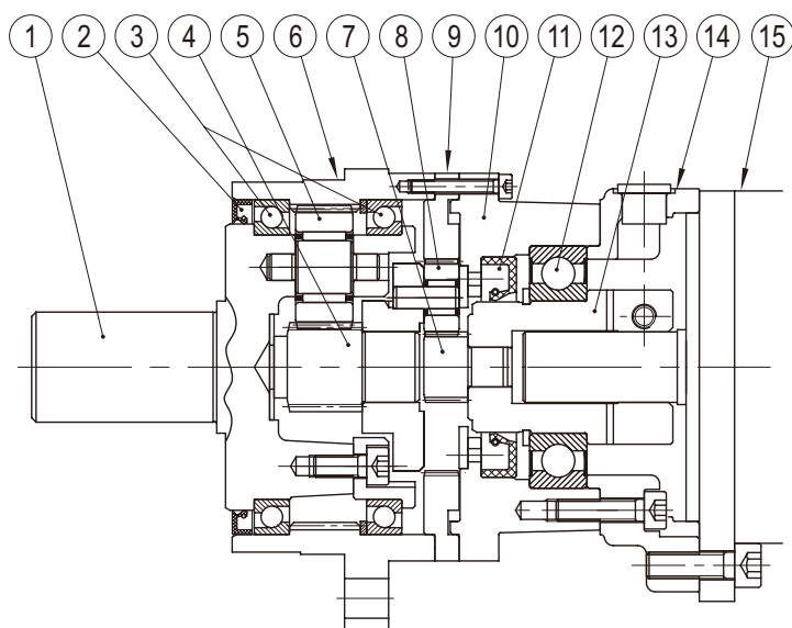
図 C1 2 段形 (例: ANFX-P120N)
