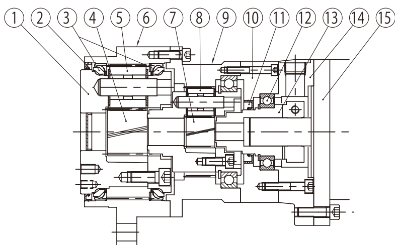
図D1 2段形 (例: ANFX-P250F)
