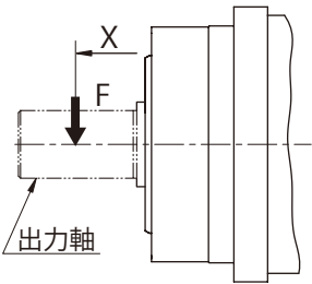
図 E3 ラジアル荷重位置
