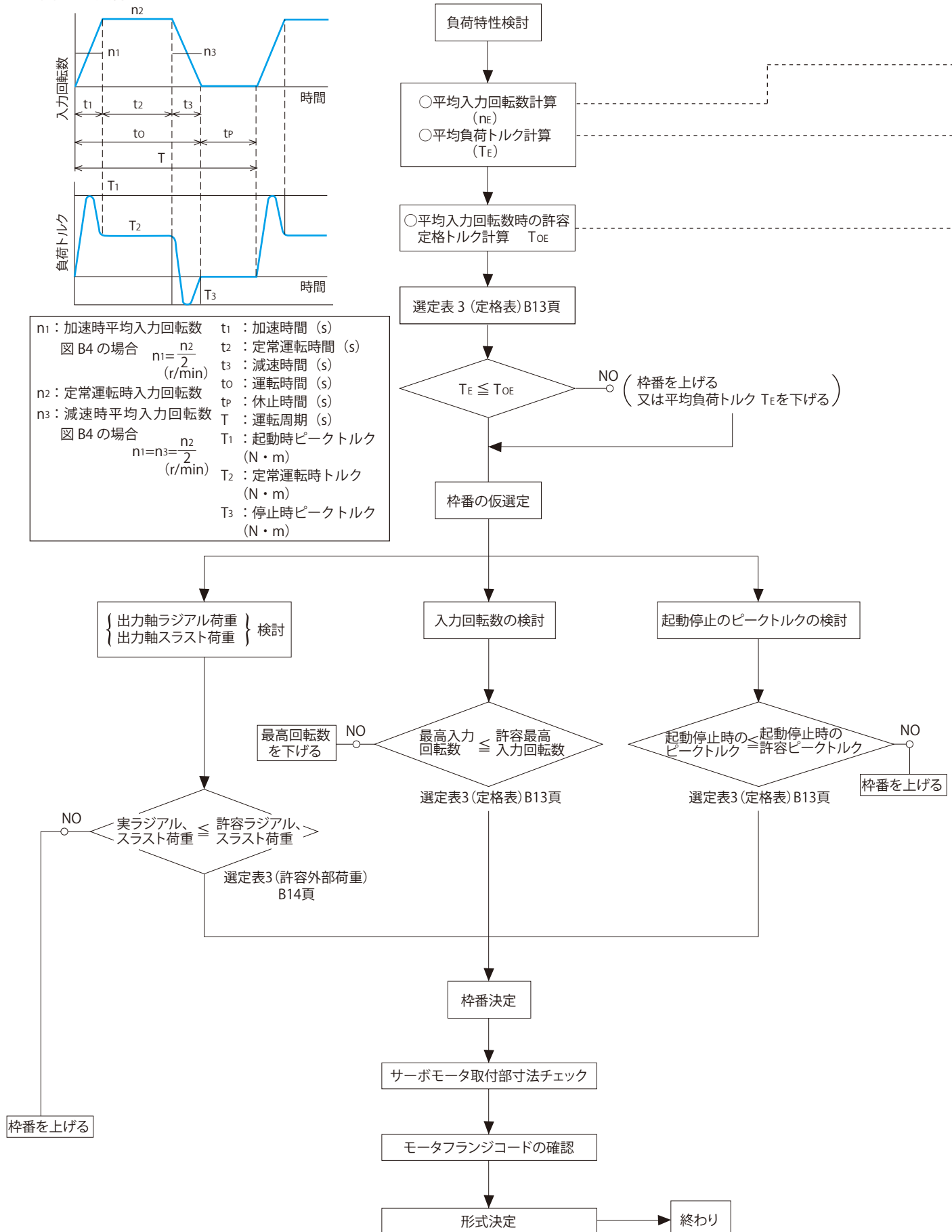
図 B4 負荷パターン
