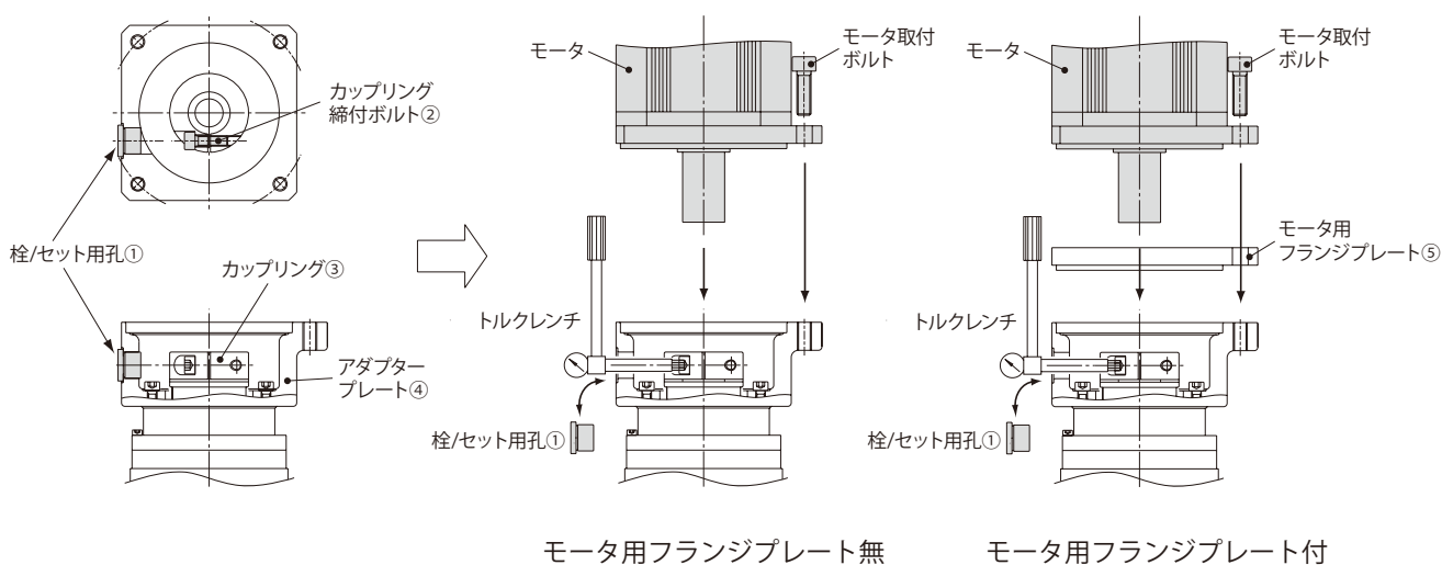
図 F2 組付図
