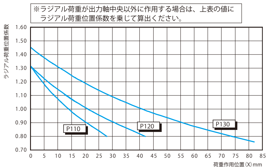
図 C2 ラジアル荷重位置係数
