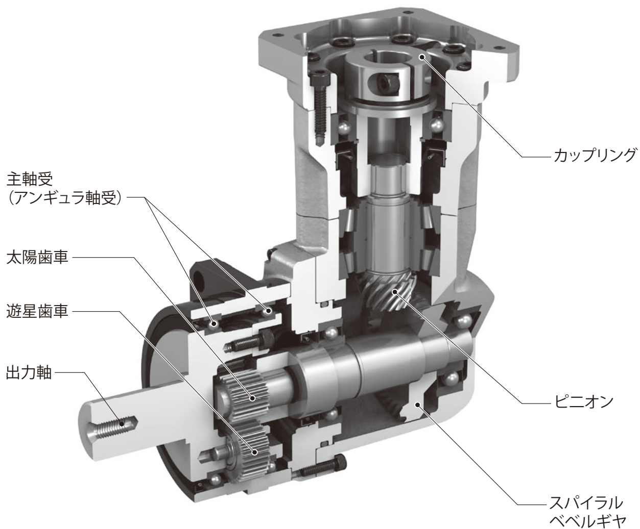
主要部品
