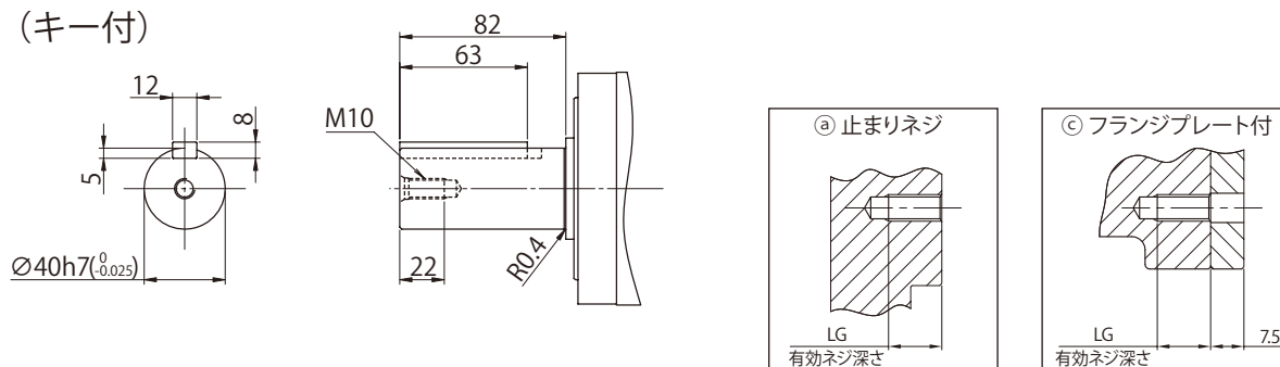
モータ取付ネジ形状詳細
