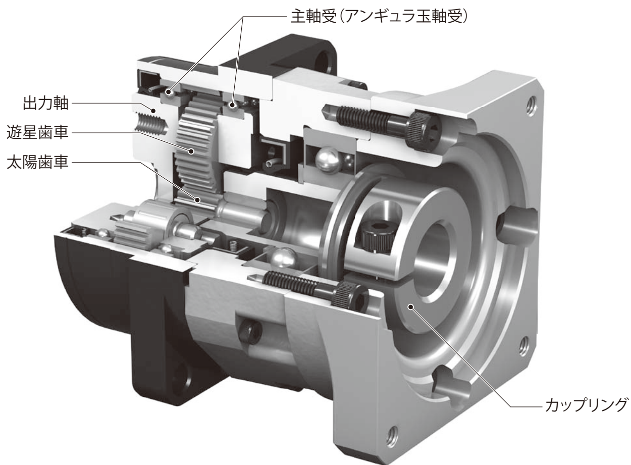
主要部品
