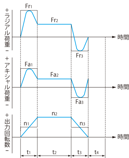
図 C6 変動荷重例
