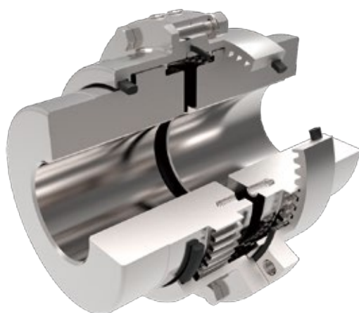
ギヤカップリング セイサGCカップリング
