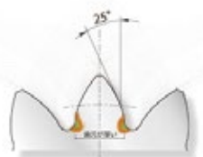
9000シリーズの歯型 (圧力角25°)
