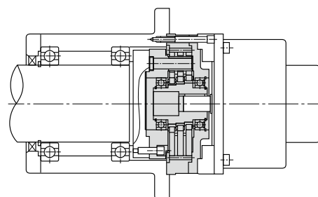
機械装置組付例
