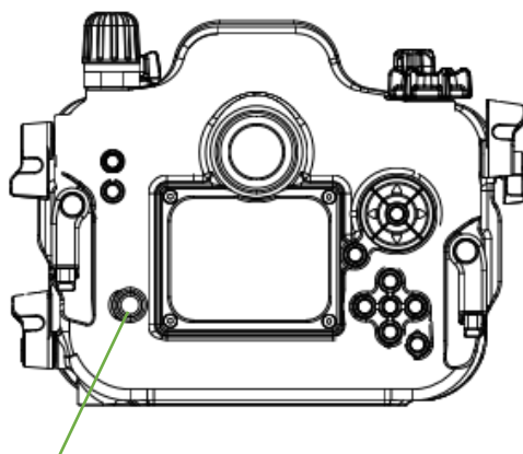
バキュームインジケータランプ
