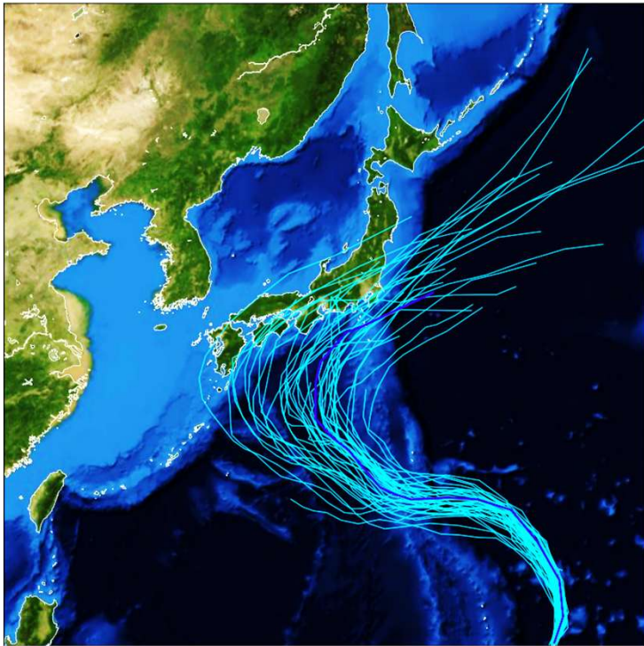
台風25号のアンサンブル予想(17日10時時点)
