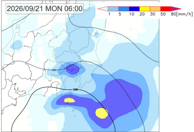
予想降水量分布図 9月21日(月)06時
