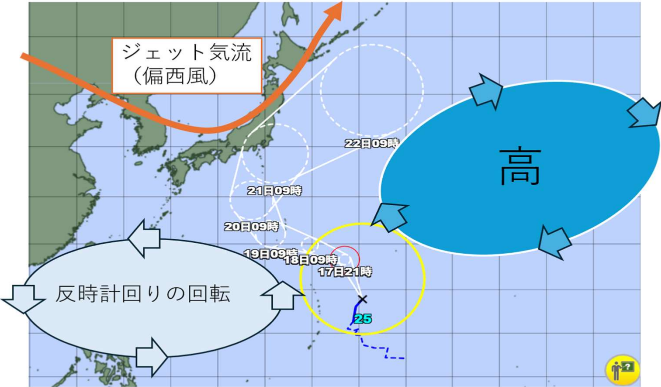
台風25号の予想進路と周辺の大気場（17日10時現在）
