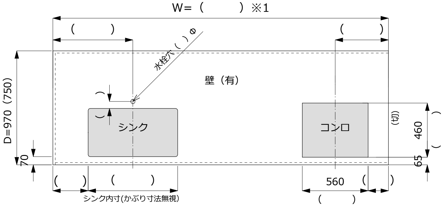
シンク勝手（図は左シンク）
