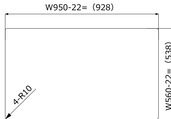
オーバーマウント参考開口寸法
