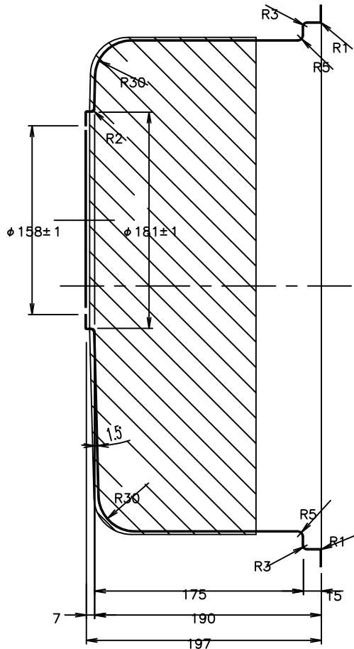
B-B 断面図(1/3)
