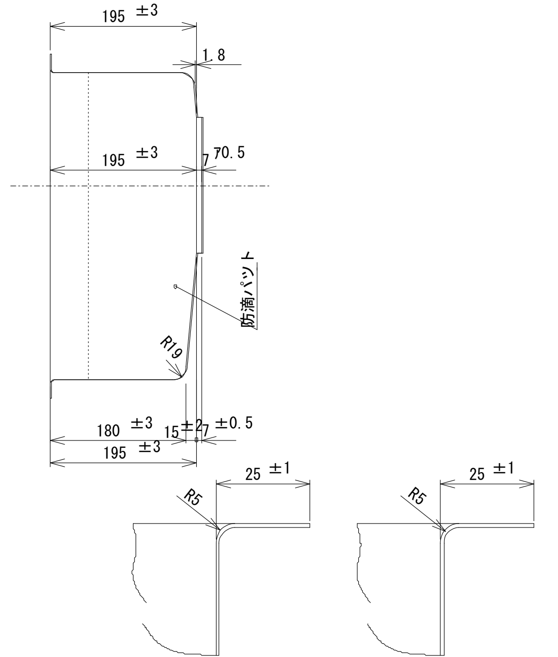
A-A' 断面 S = 1 / 1
