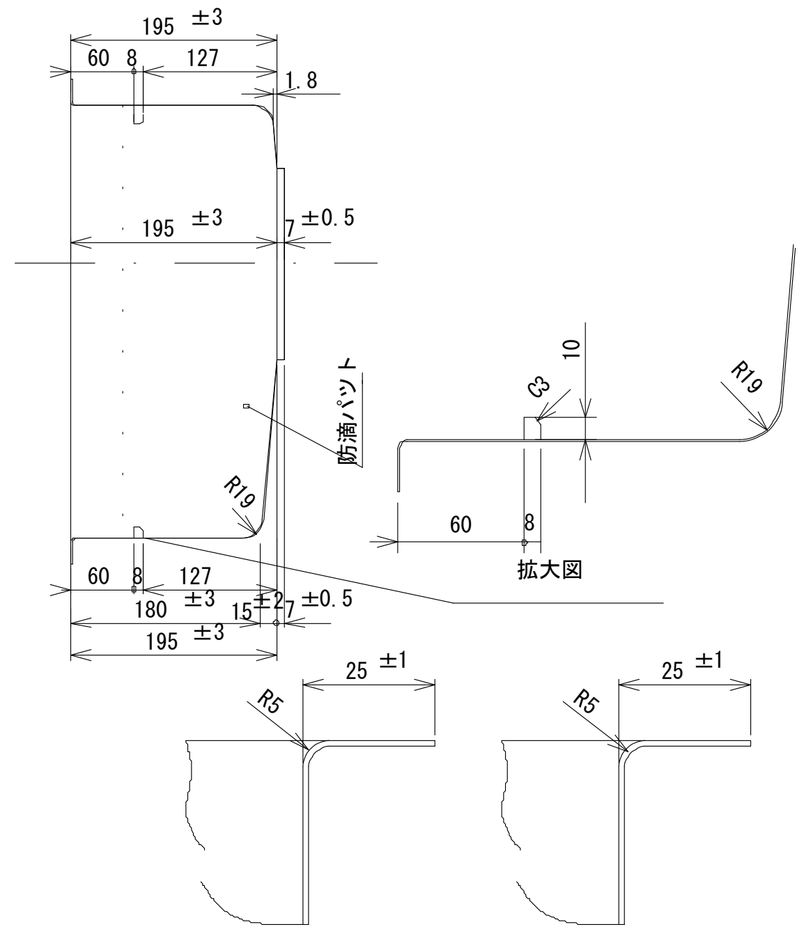
A-A' 断面 S = 1 / 1 B-B' 断面 S = 1 / 1
