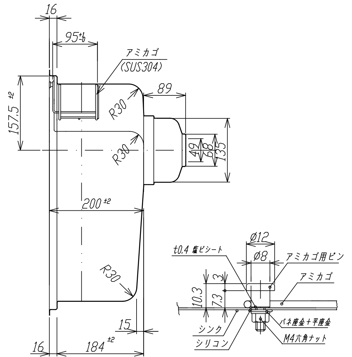
アミカゴ用ピン取付詳細 S = 1 / 1
