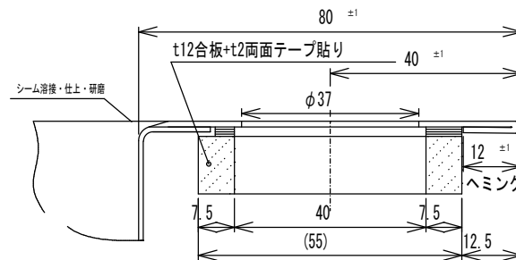
A-A' 断面 S=1/1
