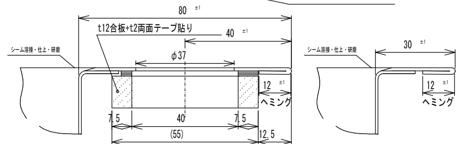
A-A' 断面 S=1/1
