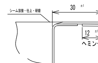
B-B' 断面 S = 1 / 1
