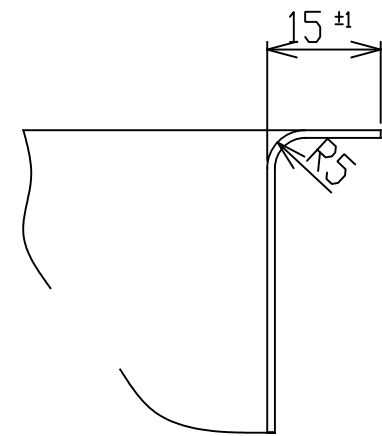
A-A'断面 S = 1 / 1
