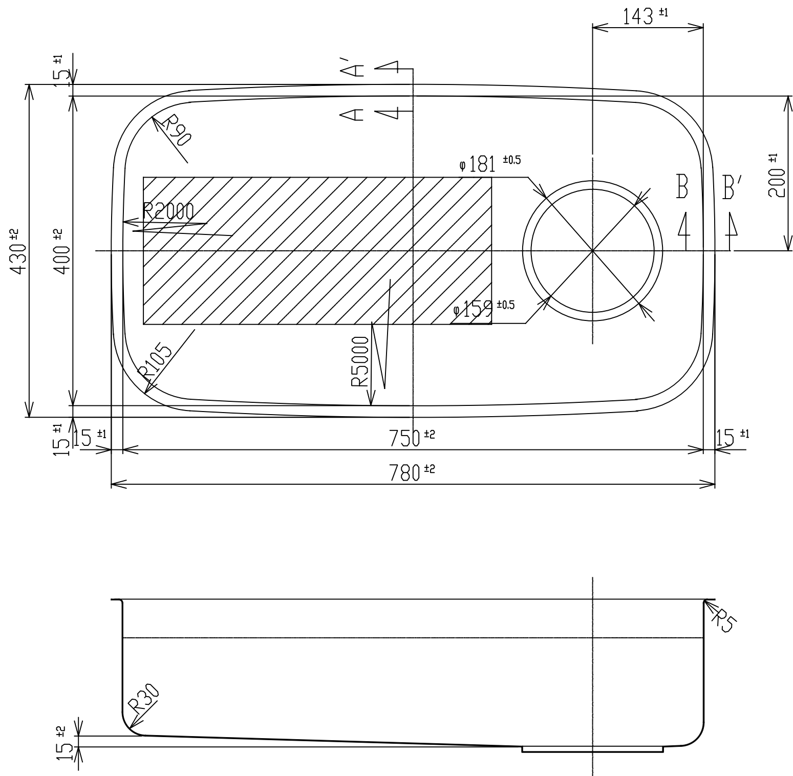
A-A'断面 S = 1 / 1
