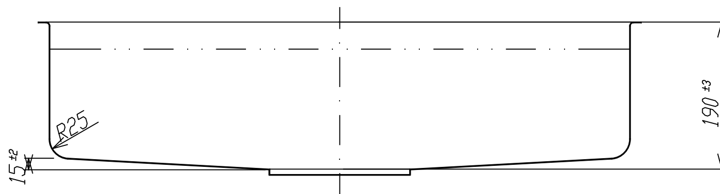
A-A'断面 S=1/1
