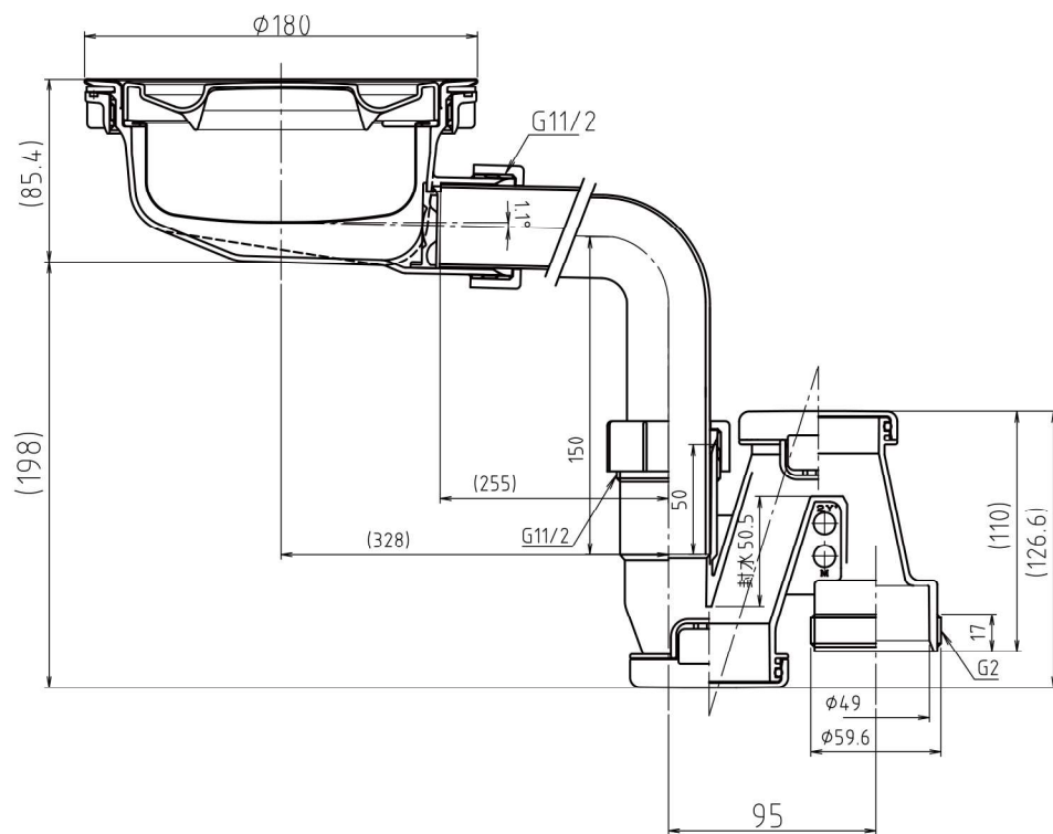
排水トラップ寸法図
