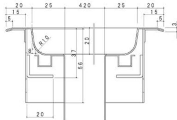
AA断面 (1/1)
