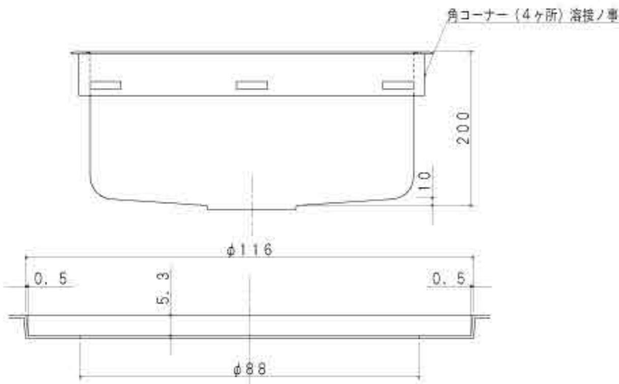
CC断面(1/1)
