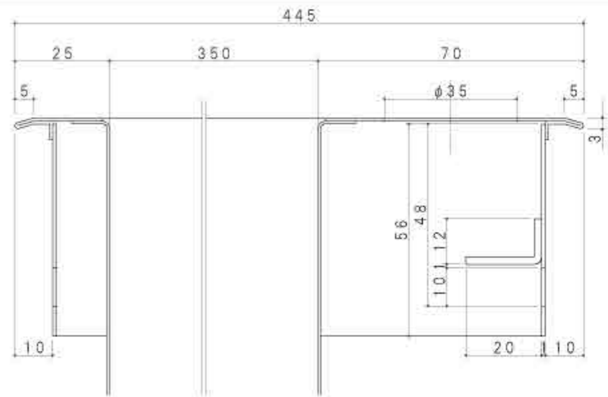
BB断面(1/1)
