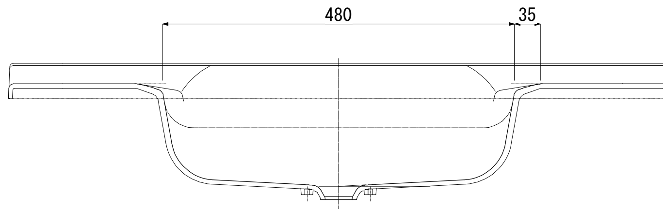
断面 B - B
