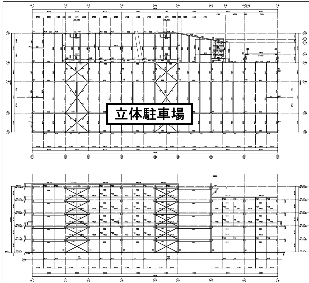
立体駐車場(2007年)
