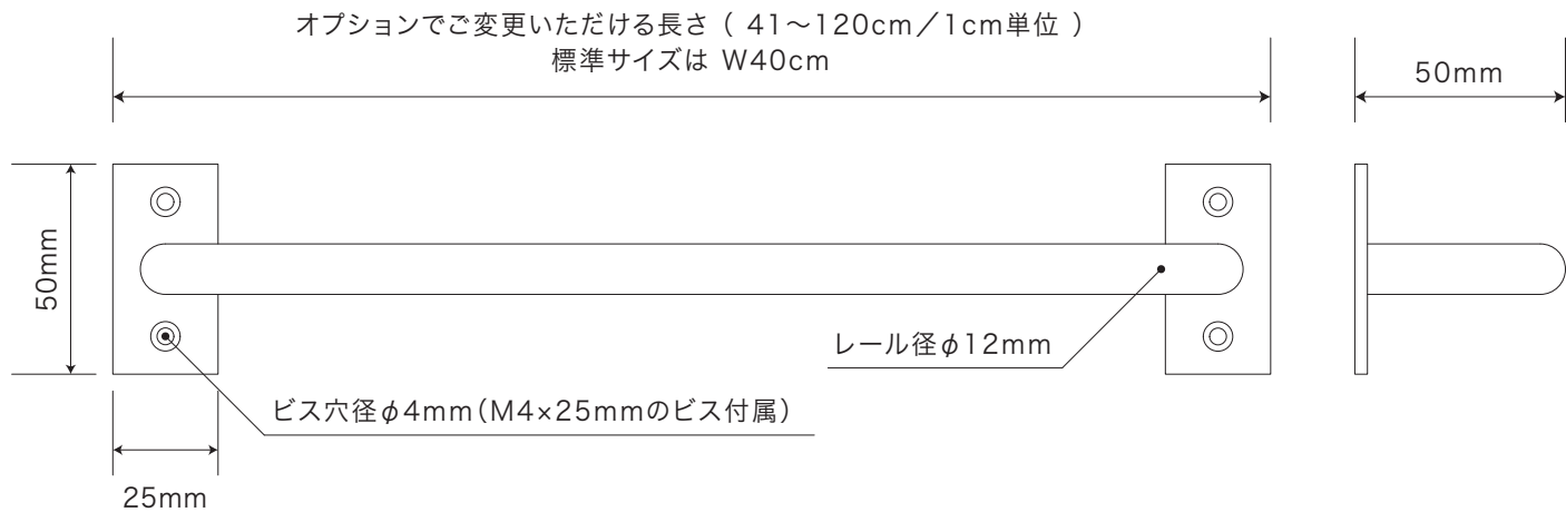
【 正 面 図 】
